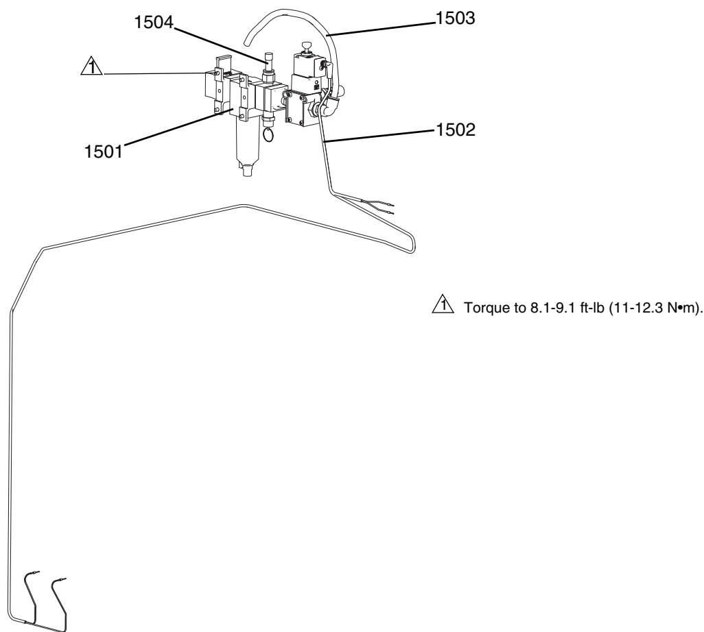
FIG. 37: Air Inlet Control
